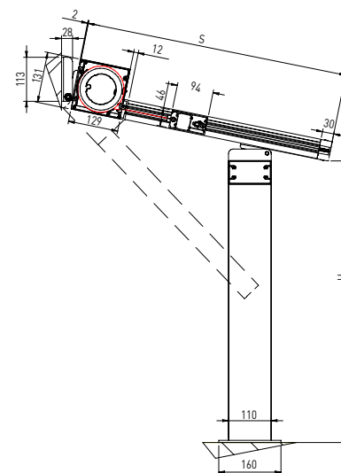
QUADRO - SQUARE A-A
